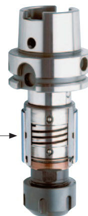
einzigartiger Flexor
