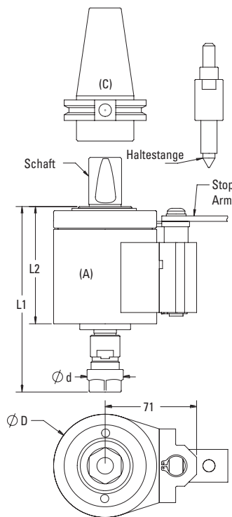
(A) Gewindeschneidapparat SPD CNC mit Zylinderschaft
