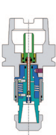
Hochdruck-Innenkühl-System
