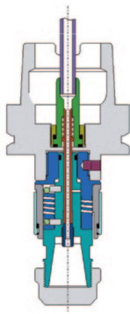
Minimalschmierungs-System
